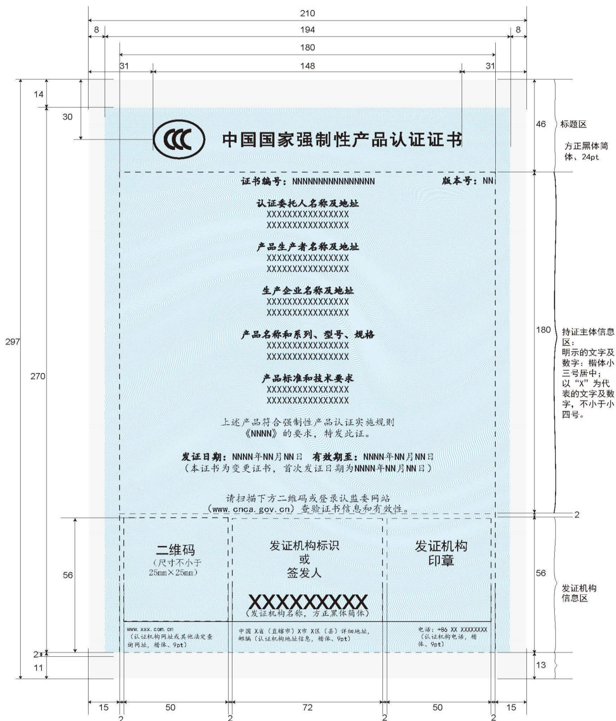
认证证书主页各功能区及规格要求（单位：mm）
